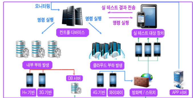
모바일 / 클라우드 / 하드웨어 부하테스트 동작 프로세스
